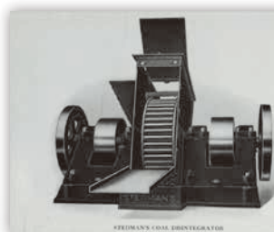
ステッドマン社の石炭破砕機
